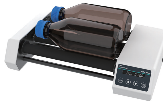
(數位顯示款)
